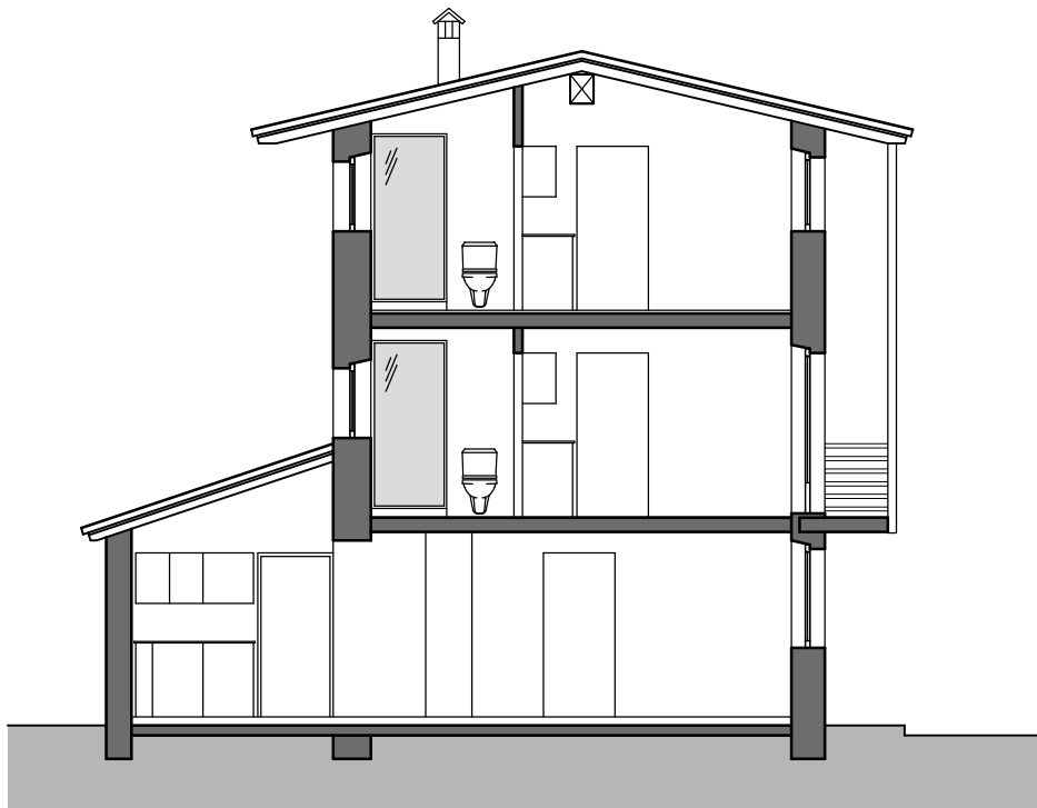
SCHNITT B-B
